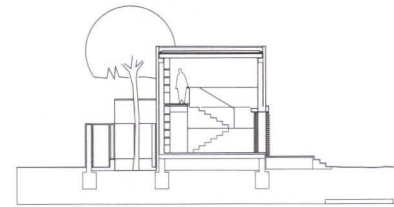
Sección por salón y galería
