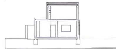
Sección por vestíbulo y despacho
