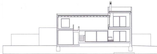
Sección longitudinal por salón
