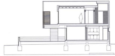
Sección por comedor y dormitorio
