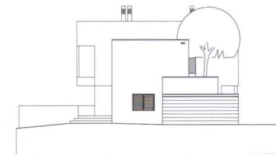
Alzado lateral
