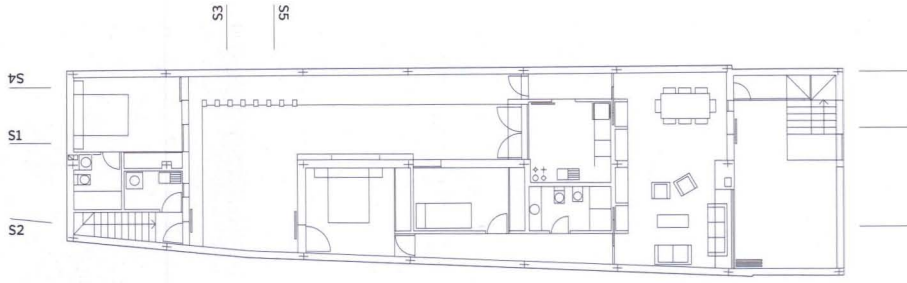
Planta baja
