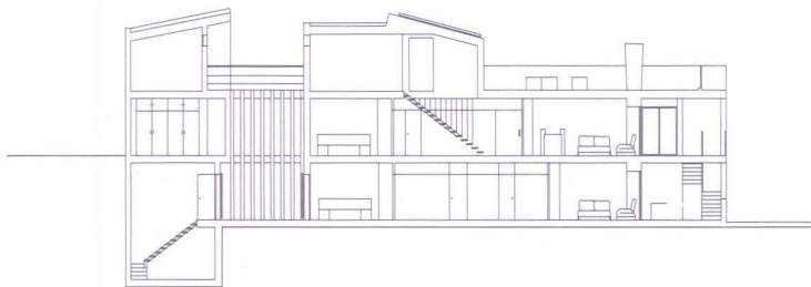
Sección S2
