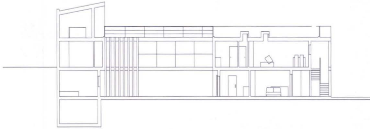
Sección S1
