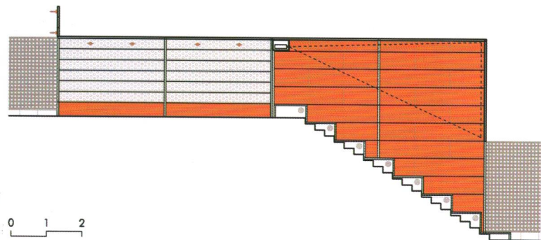
Sección longitudinal y alzados
