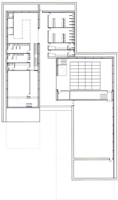
PLANTA COTA + 306.37
