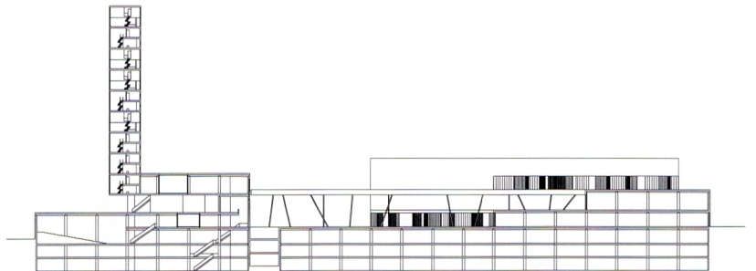
SECCIÓN B'B
