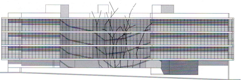
ALZADO A
