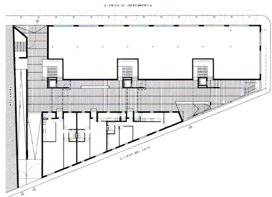
E 1:800
